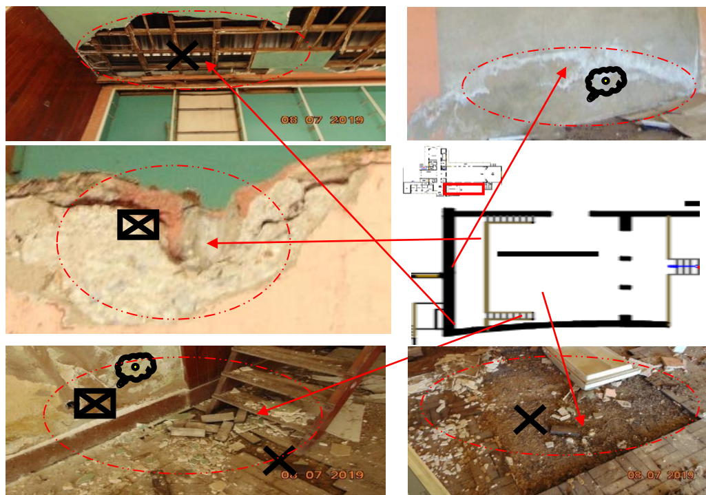
Figura 20: Alguns detalhes patológicos da sala de exposição.
