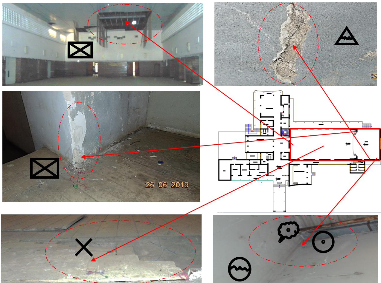
Figura 19: Alguns detalhes patológicos do edifício.
